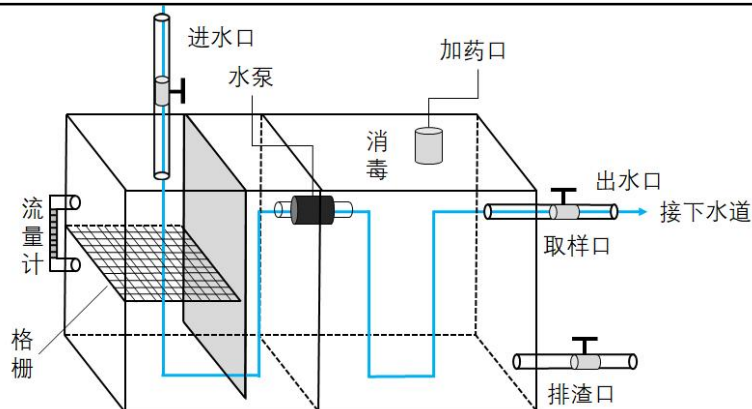
图 5 污水处理设备结构示意图
