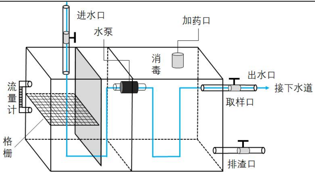
图 3 污水处理设备结构示意图
